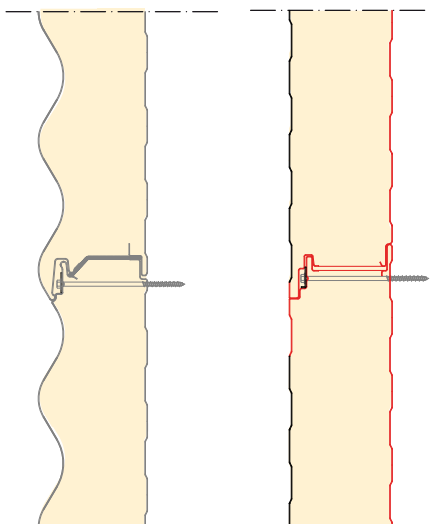
Vista in sezione Section view
