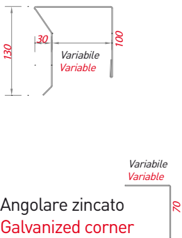
Particolare finitura superiore Superior finishing detail
