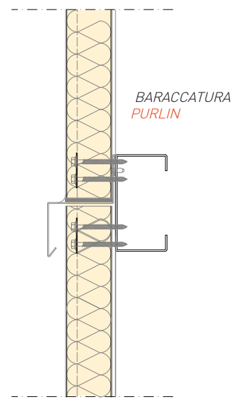
Particolare giunto di testa Head to head detail
