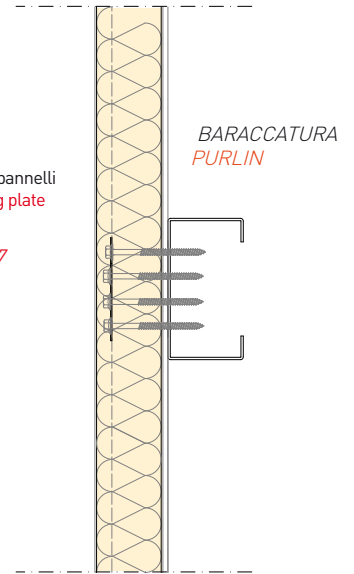
Particolare fissaggio intermedio Detail middle fixing
