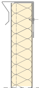
Scossalina preverniciata Cappello di finitura superiore Prepainted flashing Superior finishing cap
